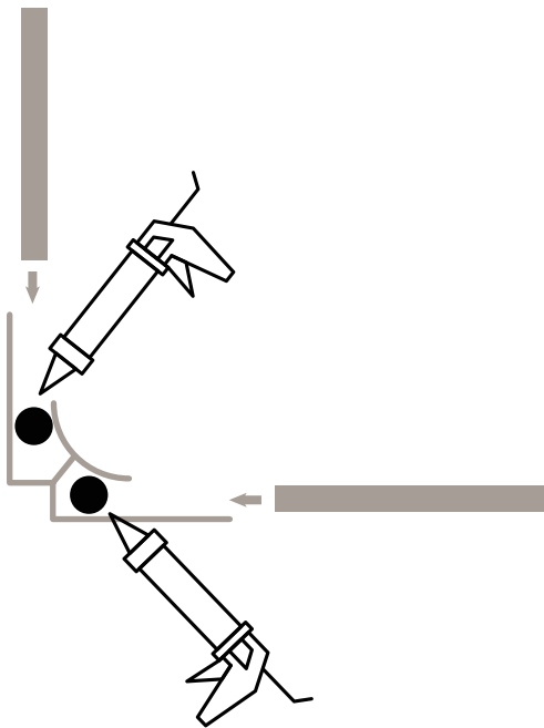
Vue de dessus profilé d'angle
